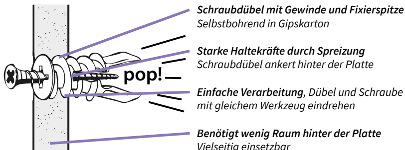
• Selbstbohrender Dübel
